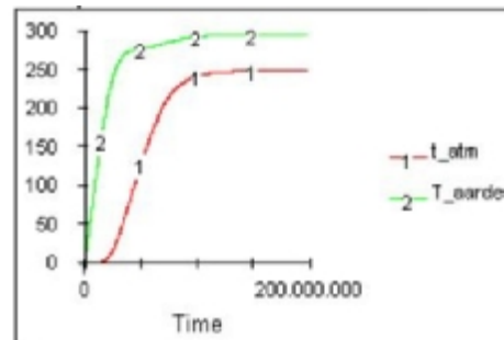
Figuur 39. Resultaat van een modelrun door II4 en II5 met het 2-laagsmodel.
