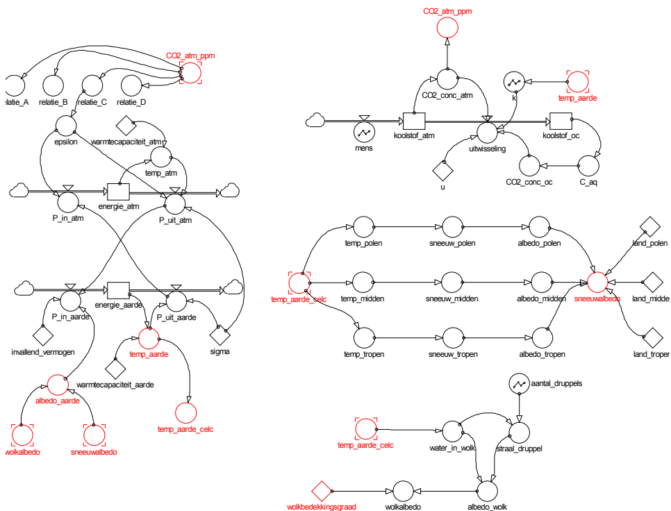
Figuur 12. Overzicht van het beoogde totaalmodel. Links het 2-laagsmodel, met bovenaan een verbinding tussen \varepsilon en een van vier mogelijke relaties met de CO 2 -concentratie. Rechts de drie specialisatiemodellen, met van boven naar beneden: oplosbaarheid van CO 2 , sneeuwbedekking in zones, en het wolkalbedo. Omwille van de duidelijkheid zijn er geen relatiepijlen getekend tussen de specialisatiemodellen en het 2-laagsmodel, hoewel het 2-laagsmodel en elk deelmodel wel modelelementen delen.
