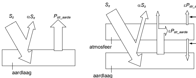
Figuur 5. Schematische weergave van het 1-laagsmodel (links) en 2-laagsmodel (rechts).
