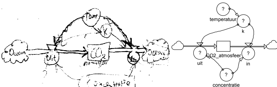
Figuur 15. Eerste schets voor het Powersimmodel van de oplosbaarheid van \text{CO}_2 in de oceaan. (Voor de duidelijkheid is rechts weergegeven hoe dit er in Powersim zou uitzien.)
