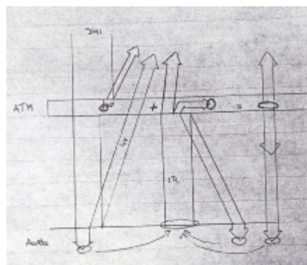
Figuur 24. Modelschets van Il4 o.b.v. de bordtekening in les 4. De labels UV en IR verwijzen naar ultraviolette en infrarode straling. De omcirkelde start- en eindpunten van pijlen duiden aan hoe de grootte van stroompijlen aan elkaar gerelateerd zijn.
