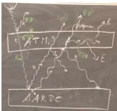
Figuur 23. Resulterende modelschets in les 3 voor de aarde met atmosfeer. R , t , a en E zijn de labels voor de processen reflectie, transmissie, absorptie en emissie. De getallen in de tekening zijn geschatte coëfficiënten voor deze processen.
