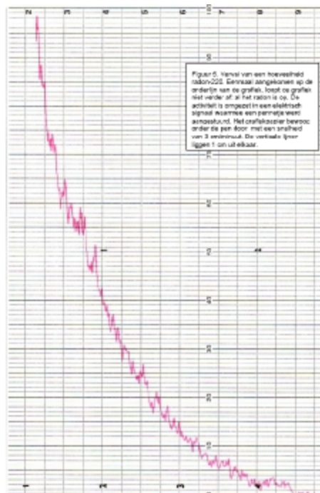
Figuur 17. Vervalgrafiek van radon-220 zoals opgenomen in het lesmateriaal.
