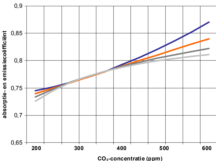
Figuur 10. Vier mogelijke relaties tussen de CO 2 -concentratie en \varepsilon . Elk leidt tot ongeveer dezelfde temperatuur voor de historische concentratieverandering sinds de Industriële Revolutie (280-380 ppm).
