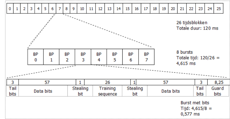
Figuur 2.12 TDMA: Tijdopdeling in blokken en bursts
