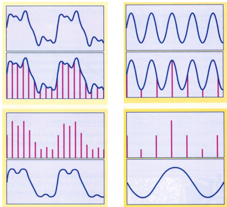
Figuur 1.16 Problemen bij te laagfrequente bemonstering. De details gaan verloren (a) en er kan een laagfrequent spooksignaal ontstaan (b).
