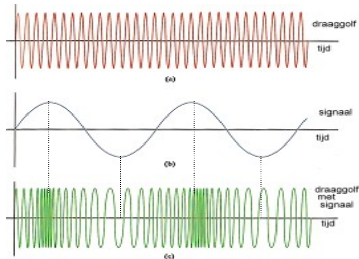
Figuur 1.8 Frequentiemodulatie. Boven (a) zien we een draaggolf als functie van de tijd, in het midden (b) zien het signaal als functie van de tijd en onder (c) zien we de draaggolf met het signaal als functie van de tijd.
