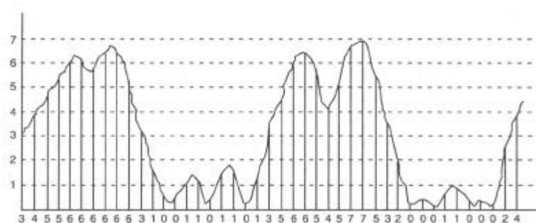
Figuur 1.18 Voor een 3-bits signaal worden alleen de waarden 0 t/m 7 toegestaan.
